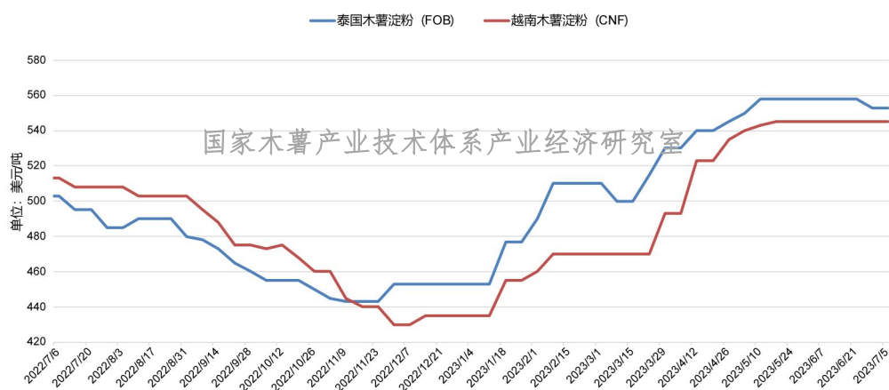
图 2 2022 年 7 月份以来泰国、越南木薯淀粉外盘价格变化情况
