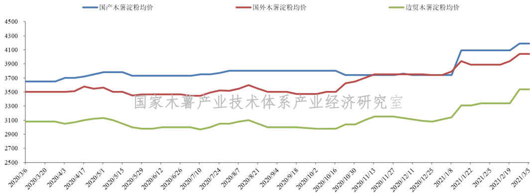
图5 2020年3月份以来中国各类木薯淀粉均价变化情况 单位: 元/t
