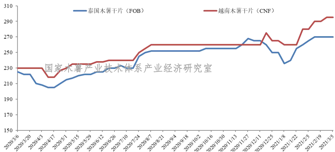
图3 2020年3月份以来泰国、越南木薯干片价格变化情况 单位：美元/t
